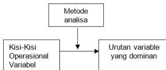
Gambar 2. Tahapan Penelitian
