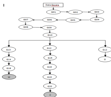
Gambar 2. Diagram Keputusan Sistem Pakar
