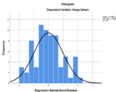
(Sumber: SPSS versi 25, 2020) Gambar 2 Histogram
